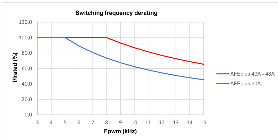
FIG. 7 - Declassamento frequenza di switching / Switching frequency derating
