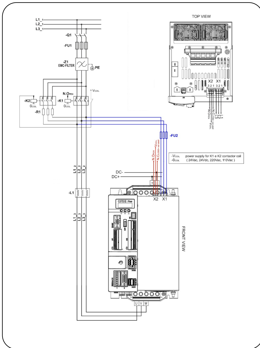
FIG. 22- Connessione alla rete dell'FFE / FFE Main connection
