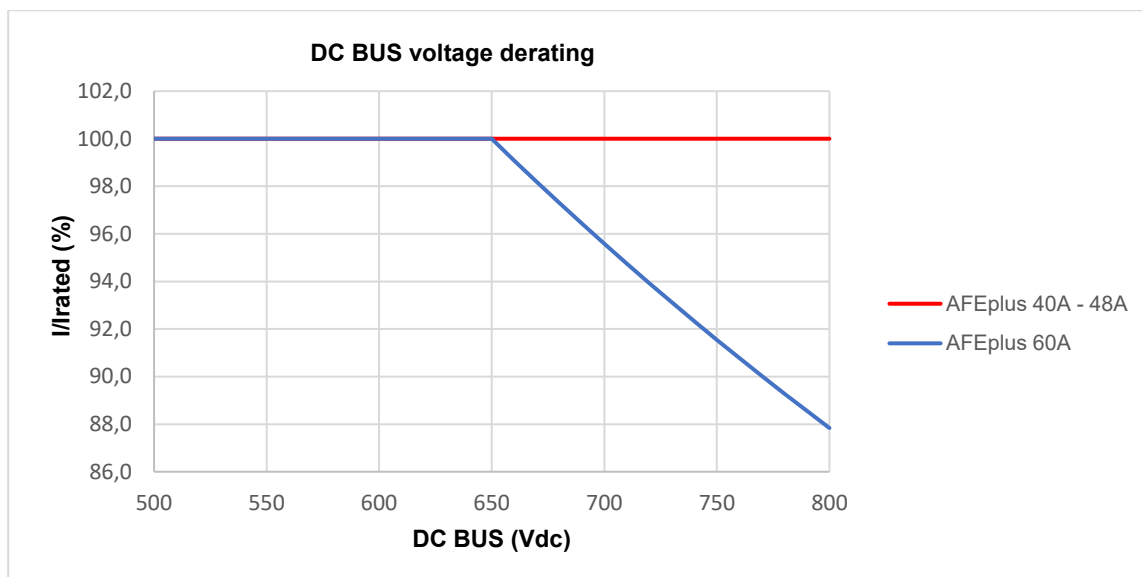
FIG. 4 - Declassamento tensione d'ingresso / Input voltage derating
