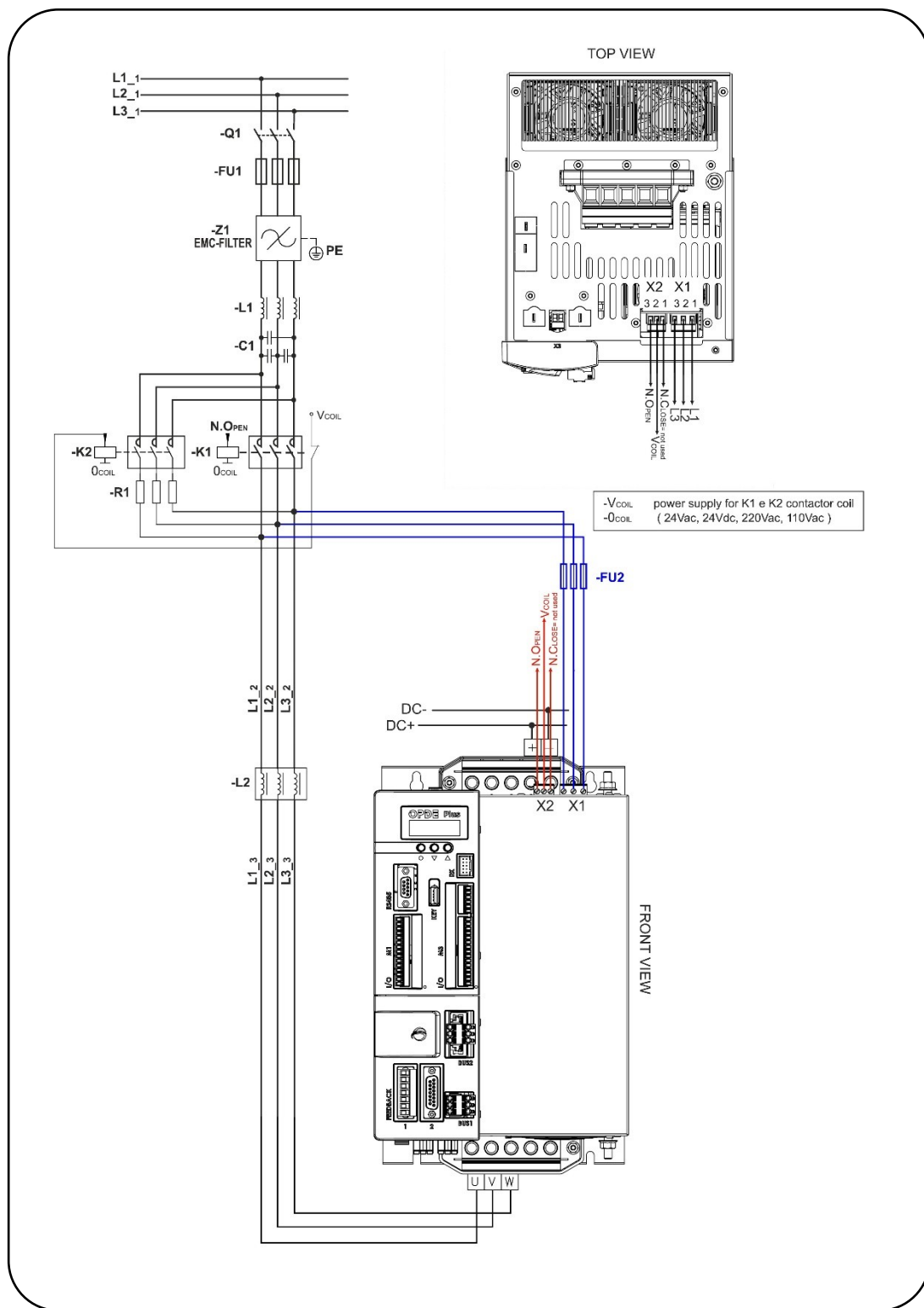
FIG. 14-Connessione alla rete dell'AFEplus / AFEplus Main connection
